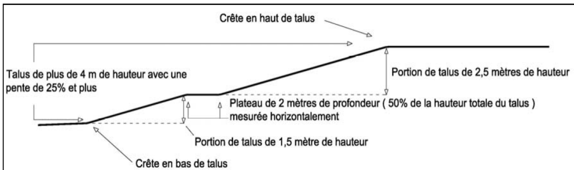
Illustration d'un talus de 4 mètres de hauteur, entrecoupé d'un plateau de 2 mètres et plus de profondeur, où les normes relatives aux secteurs de forte pente ne s'appliquent pas.
