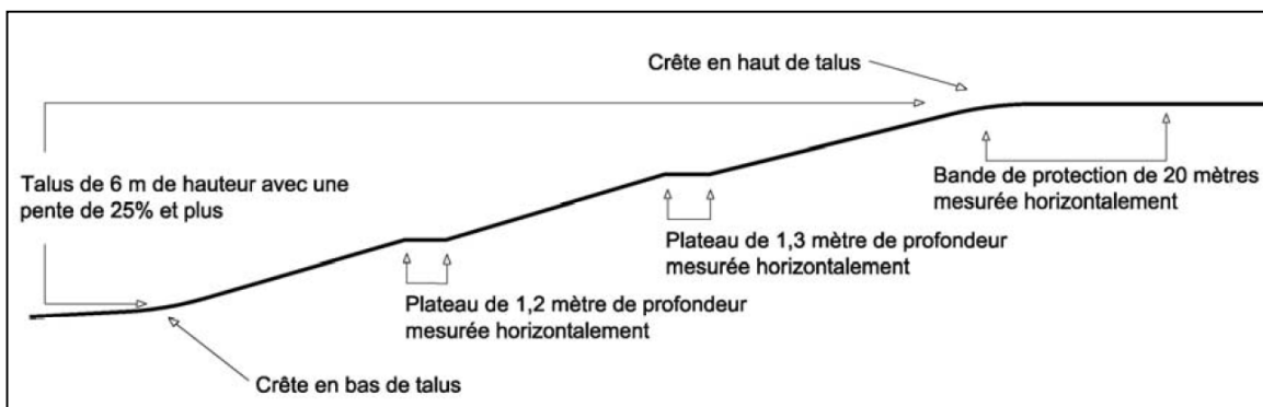
Illustration d'un talus de 6 mètres de hauteur, entrecoupé de deux plateaux de 1,2 mètre et de 1,3 mètre de profondeur et qui ne dépassent pas 40 % de la hauteur totale du talus : les normes relatives aux secteurs de forte pente s'appliquent.
